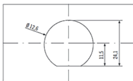
Frontplattenausschnitt
